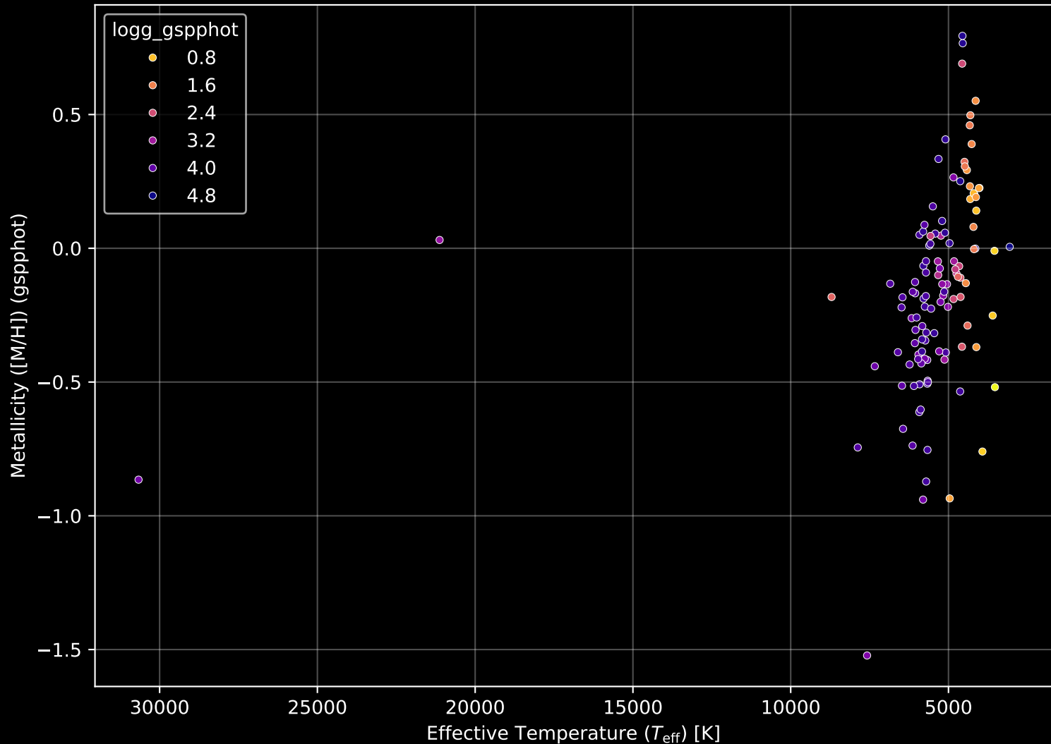
APOGEE DR17 Field: [279-36-O_TESS] Stellar Population Parameters (n= 117)
